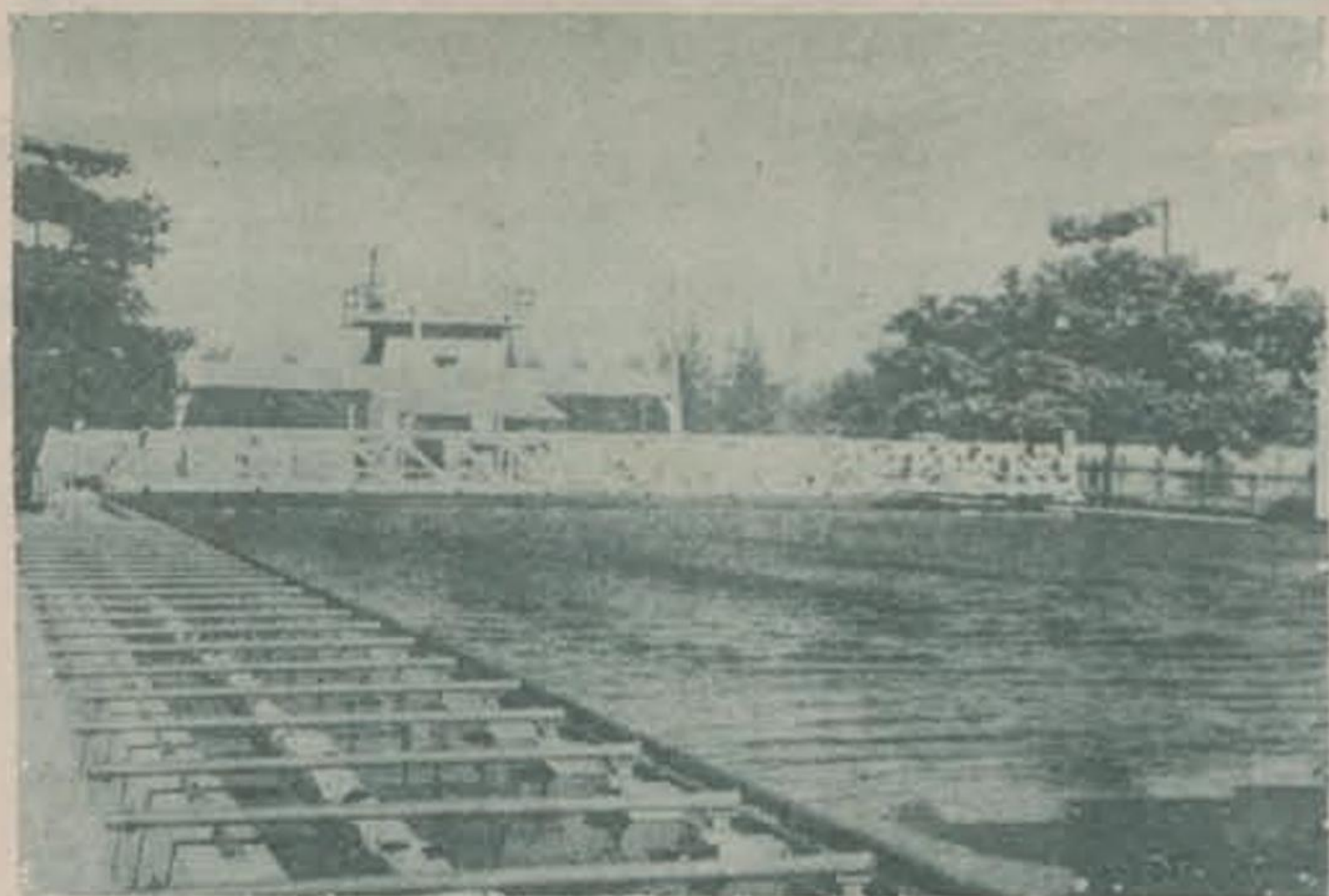
↑ 工學院土木系及水利系與基隆港務局在建教合作之契約下，接受委託作臺中港之沙粒移動試驗及各種防沙堤之試驗，圖為平面規形之全景。
